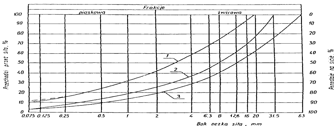
Rysunek1. Pole dobrego uziarnienia kruszyw przeznaczonych na podbudowy wykonywane metodą stabilizacji mechanicznej 1-2 kruszywo na podbudowę zasadniczą (górną warstwę) lub podbudowę jednowarstwową 1-3 kruszywo na podbudowę pomocniczą (dolną warstwę)
