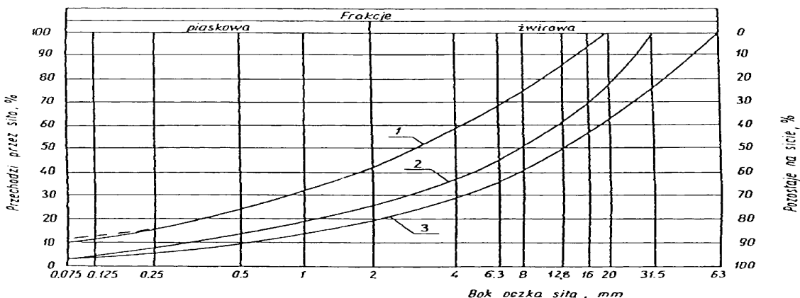
Rysunek1. Pole dobrego uziarnienia kruszyw przeznaczonych na podbudowy wykonywane metodą stabilizacji mechanicznej 1-2 kruszywo na podbudowę zasadniczą (górną warstwę) lub podbudowę jednowarstwową 1-3 kruszywo na podbudowę pomocniczą (dolną warstwę)
